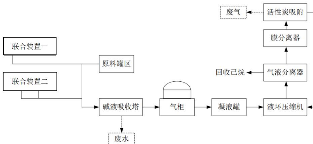
图 12 废气处理工艺流程图
