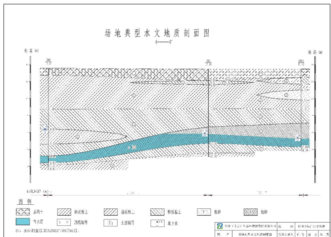
图 7 厂区地层剖面图 (4-4' )
