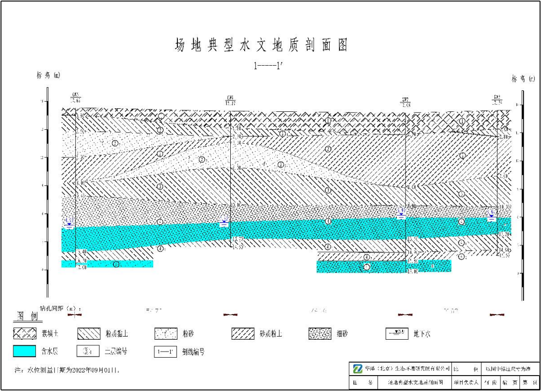
图 4 厂区地层剖面图 (1-1' )
