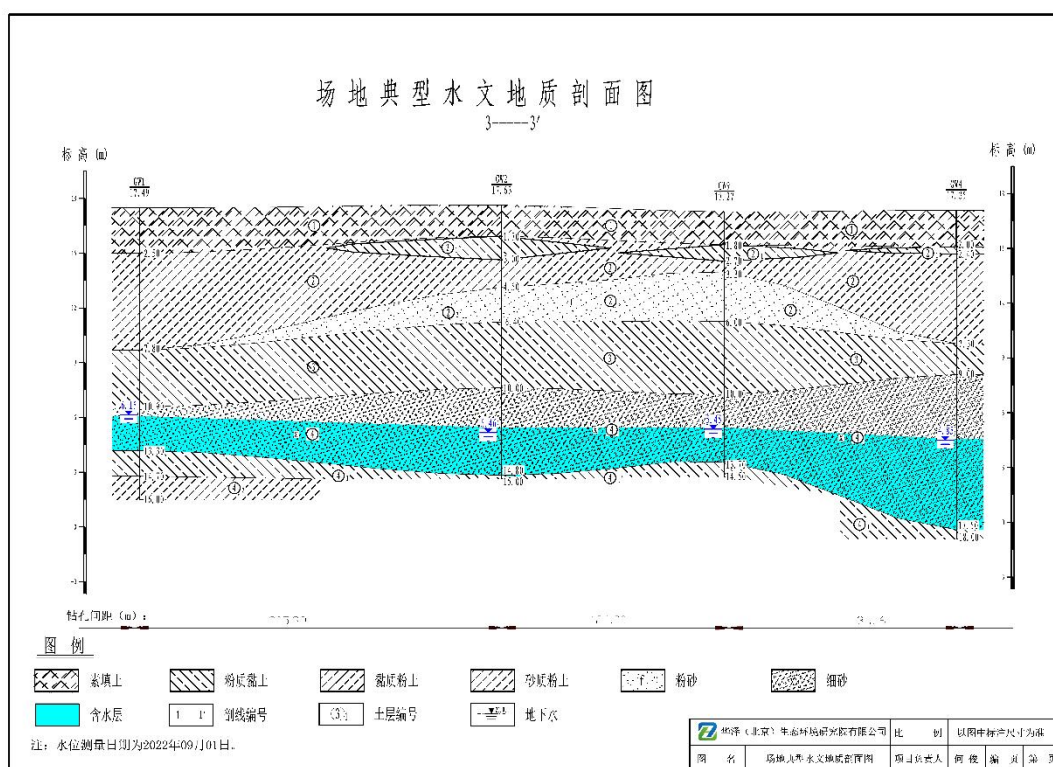
图 6 厂区地层剖面图 (3-3' )
