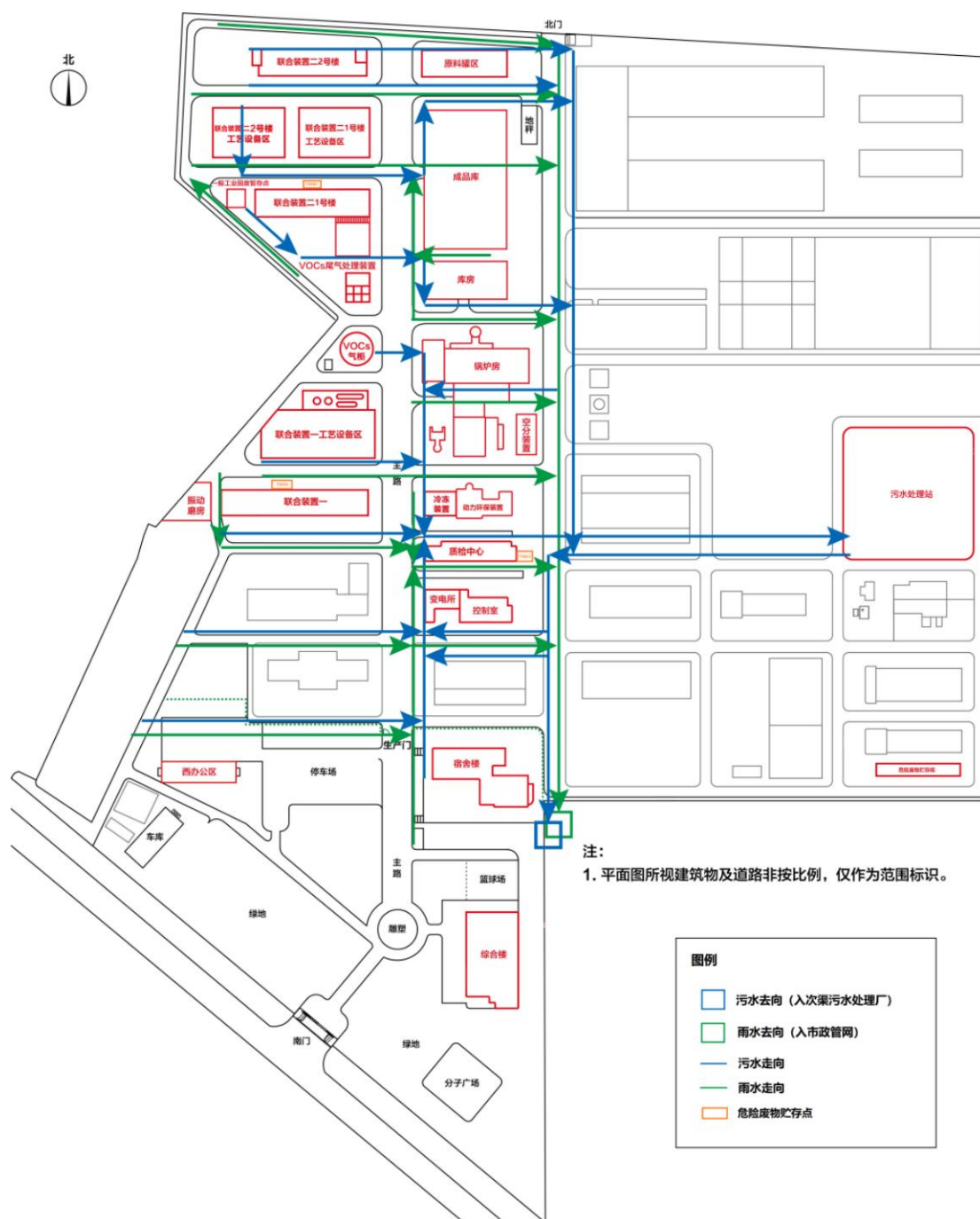
图 10 企业雨污管线图
