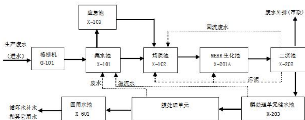
图 13 废水处理工艺流程图
