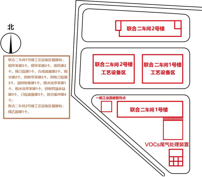
图 18 联合二车间储罐分布图
