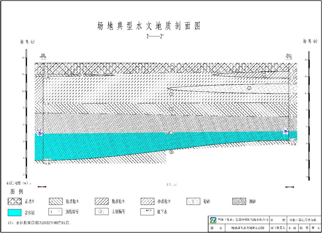
图 5 厂区地层剖面图 (2-2' )
