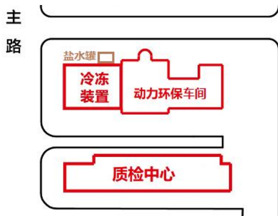
图 19 动力环保车间储罐分布图
